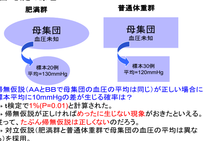
図 検定の原理
